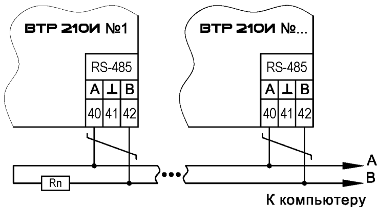
Рисунок 4.2 - Схема подключения ПК к блоку ВТР с интерфейсом RS-485
