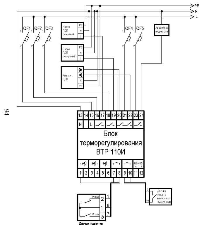
Рисунок В.3-Схема подключения регулятора ВТР 110И (программа 40) в системе управления контуром подпитки
