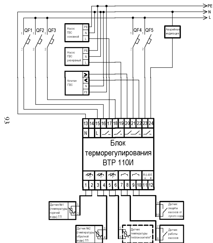
Рисунок В.2-Схема подключения регулятора ВТР 110И (программа 20) в системе управления контуром ГВС
