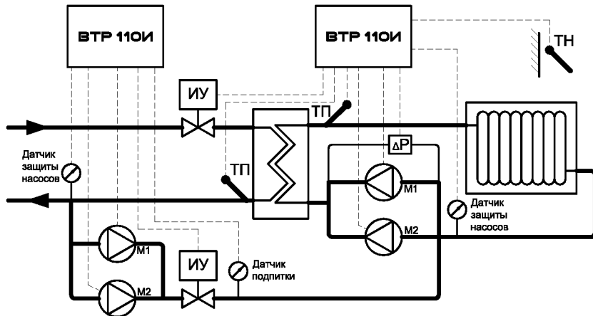
Рисунок Б.2 – Монтажная схема регуляторов ВТР 110И в системе управления независимым контуром отопления (программа 10) и контуром подпитки (программа 40)
