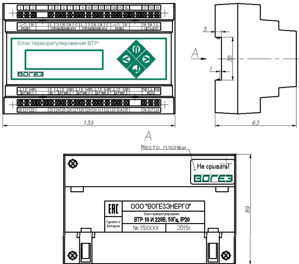
Рисунок А.1 Габаритные и установочные размеры блока терморегулирования ВТР-10И
