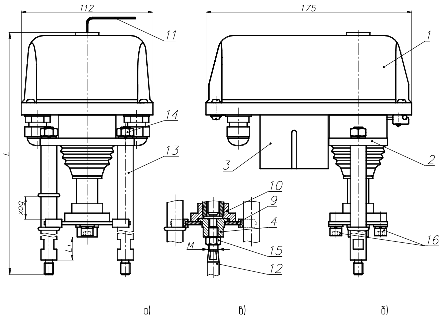
Рисунок 1. ВЭП-12Х
